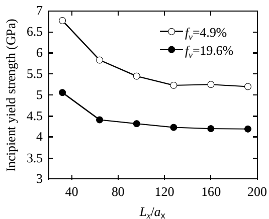
Fig.2 [\bar{1}10]-[111]-[11\bar{2}] case
