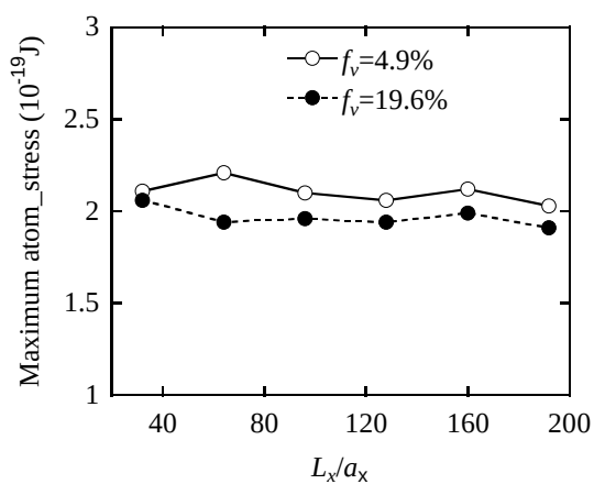
Fig.4 [\bar{1}10]-[111]-[11\bar{2}] case
