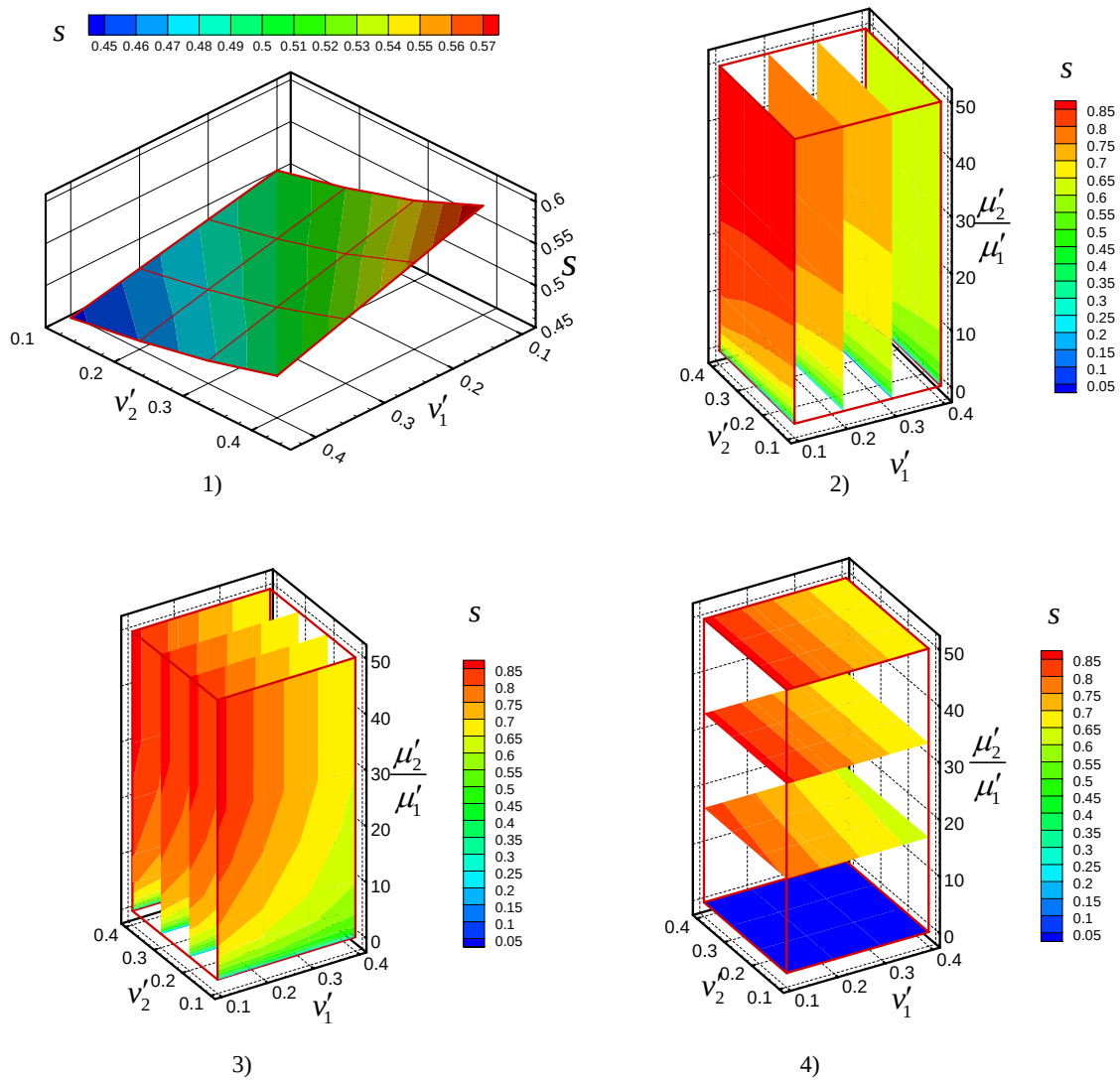
图 5-2 裂纹前沿广义应力奇性指数随材料参数变化规律
